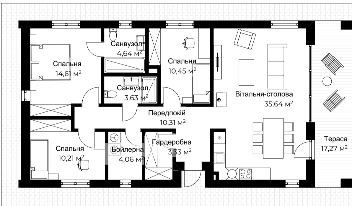
ПЛАН ПОВЕРХУ
